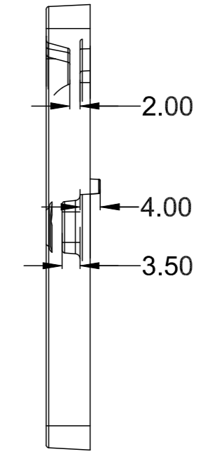
截面 A-A
